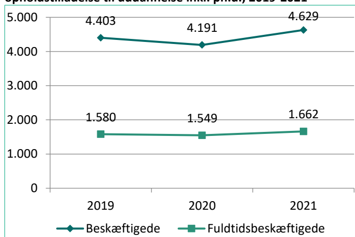
Figur 13.1 – Antal beskæftigede og fuldtidsbeskæftigede med opholdstilladelse til uddannelse inkl. ph.d., 2019-2021
